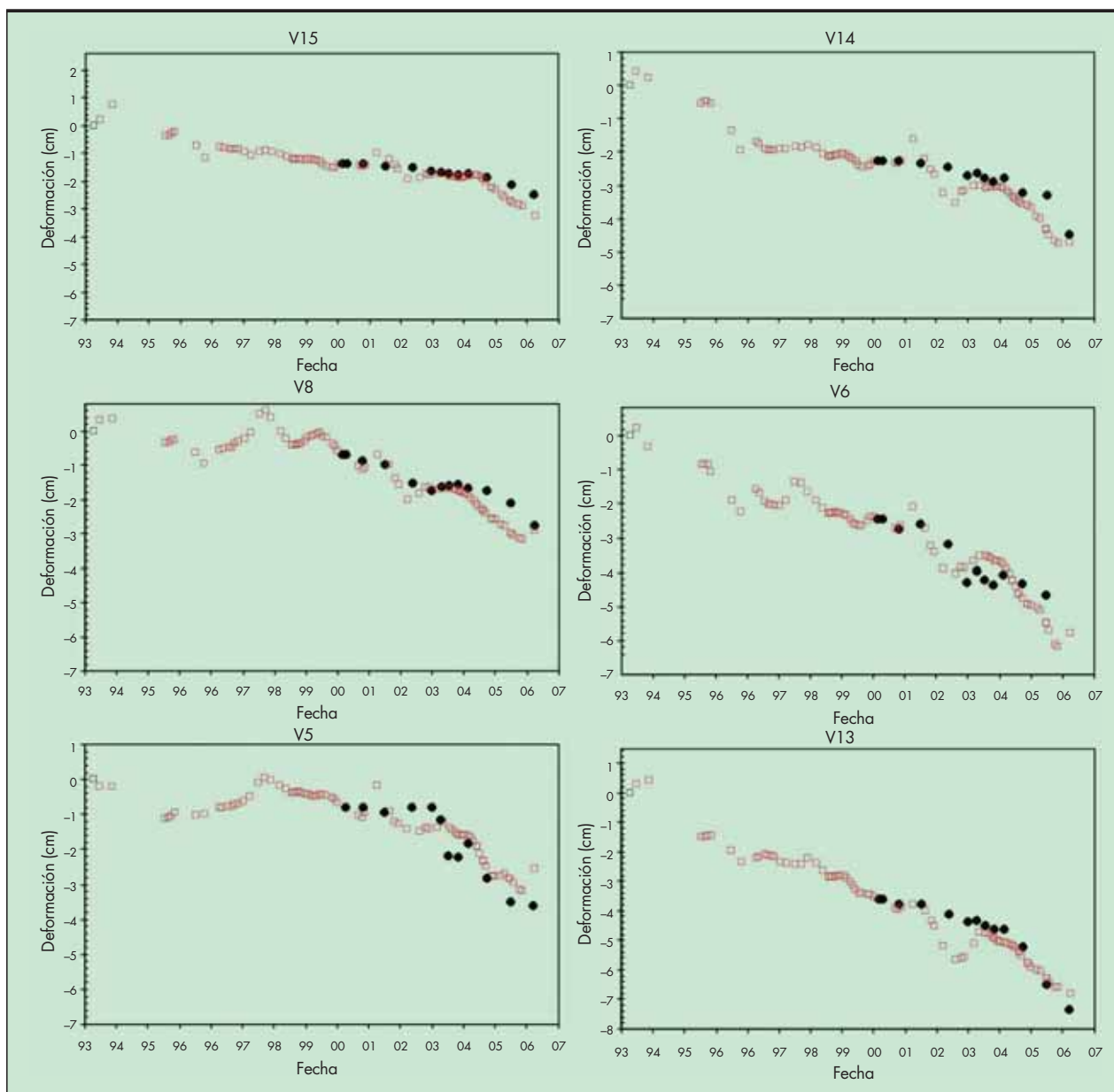
FIGURA 7. Superposición de los datos de subsidencia medidos con los extensómetros (puntos) y la interferometría SAR diferencial (cuadrados).
